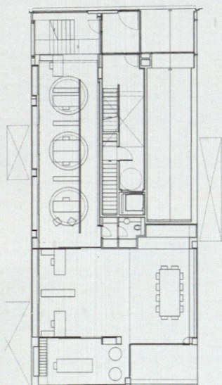
03 - PLANTA PRIMERA
