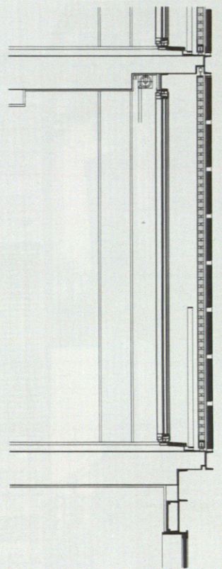
08 - SECCIÓN CERRAMIENTO
