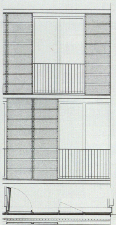
07 - ALZADO TIPO Y PLANTA
