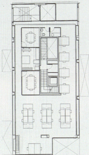
04 - PLANTA SEGUNDA
