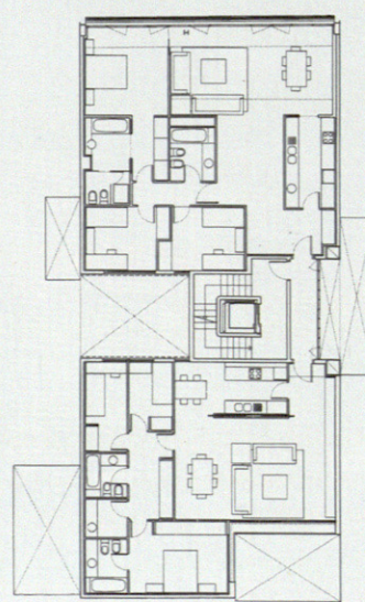
06 - PLANTA CUARTA
